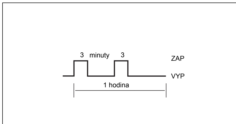
Obr. 10 Znárodnění doby chodu cirkulačního čerpadla s nastavením od výrobce 2
