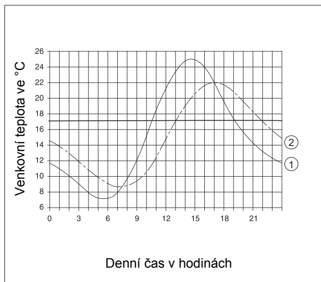
Obr. 7 Průběh teplot
