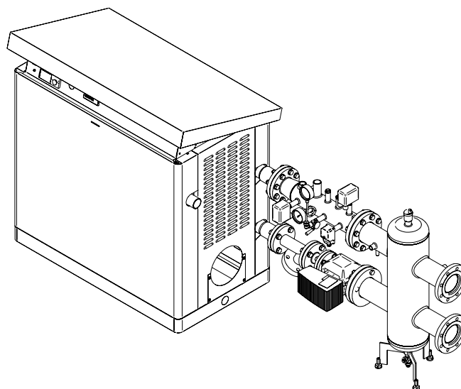
Krycí sada pro venkovní soupravy s hydraulickým oddělovačem.
