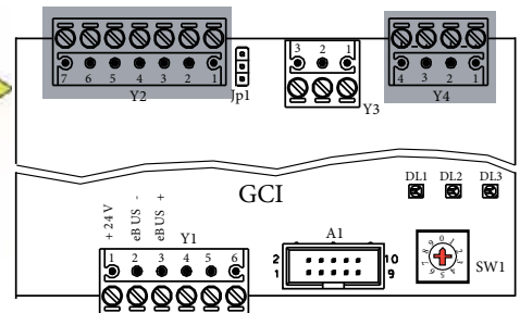
Svorkovnice GCI (zadní strana)
