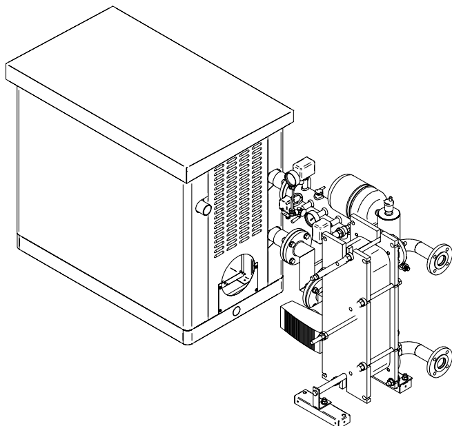
Krycí sada pro venkovní soupravy s deskovým výměníkem tepla.
