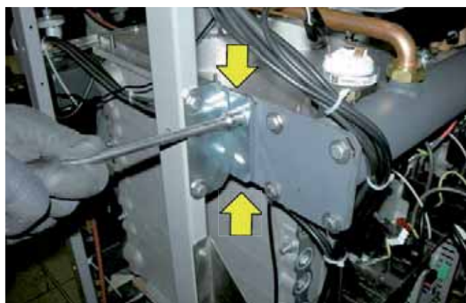
- Odstraňte šrouby upevňující plynovou trubku (pravá a levá strana).
