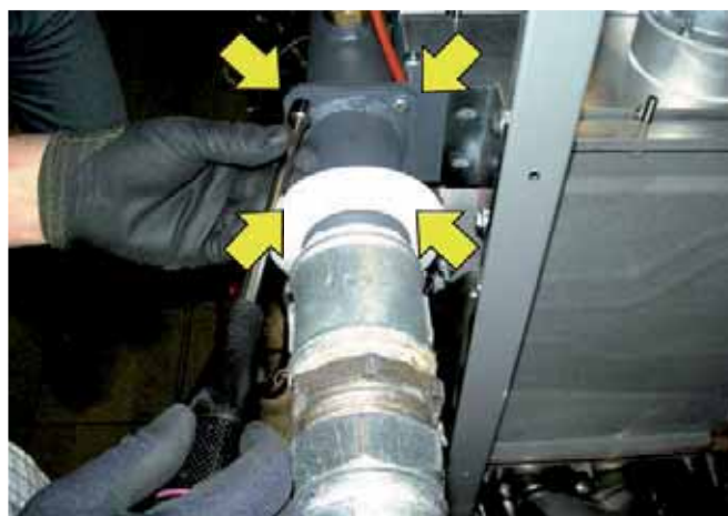
- Odstraňte čtyři šrouby trubkovým klíčem 10 mm, pak přírubu plynu.
