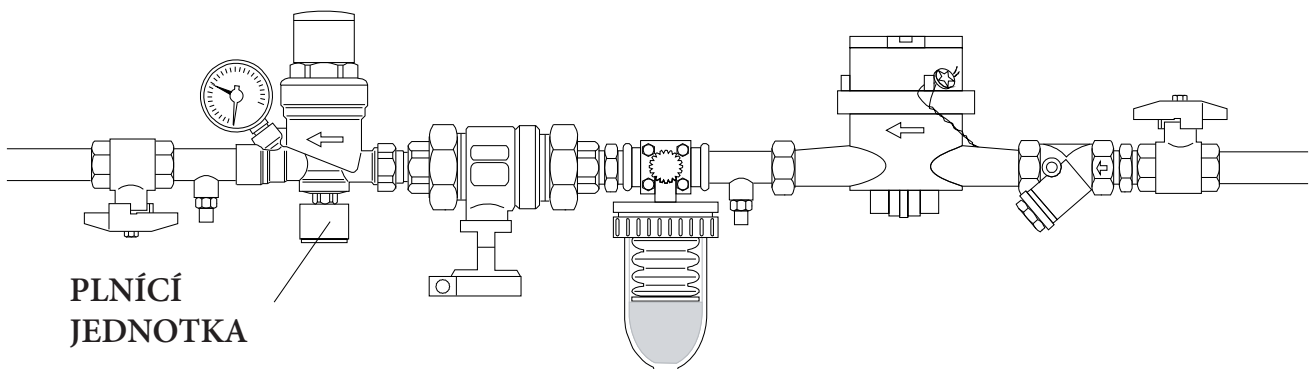
PŘÍKLAD PLNÍČÍ JEDNOTKY ZAŘÍZENÍ
