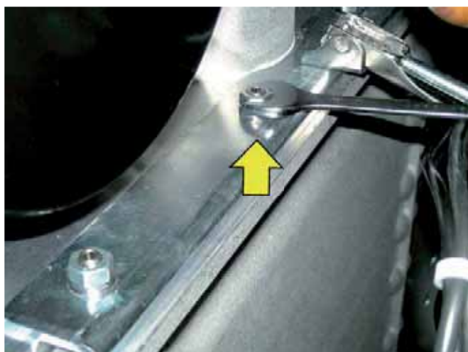
- Odstraňte šrouby "B" (trubkovým klíčem 13 mm / šestihránným klíčem 13 mm) a odstraňte plechové upevňující podložky.
