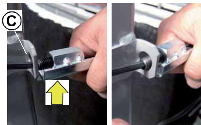
- Jemně nadzvedněte zadní blok hořáků a vytáhněte 2 čepy pomocí šestihranného klíče 5 mm, až dokud nedosáhnete na otvory "C" (levá a pravá strana).
