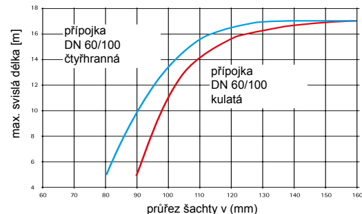
kouřovod DN 60
