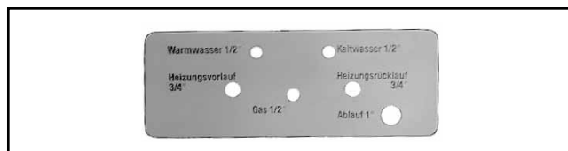
Obr: Montážní šablona pod omítkou
