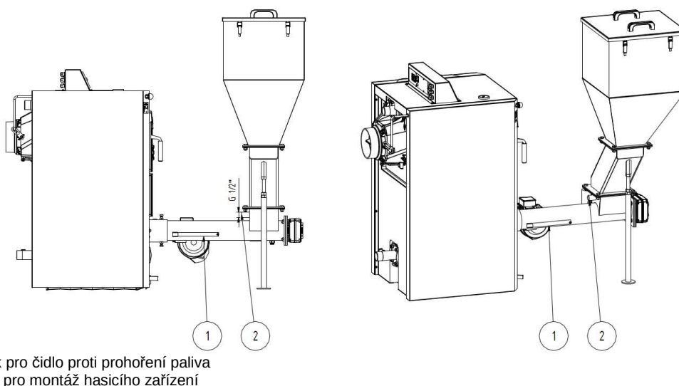
Obr. č. 24 Montáž havarijního hasicího zařízení
