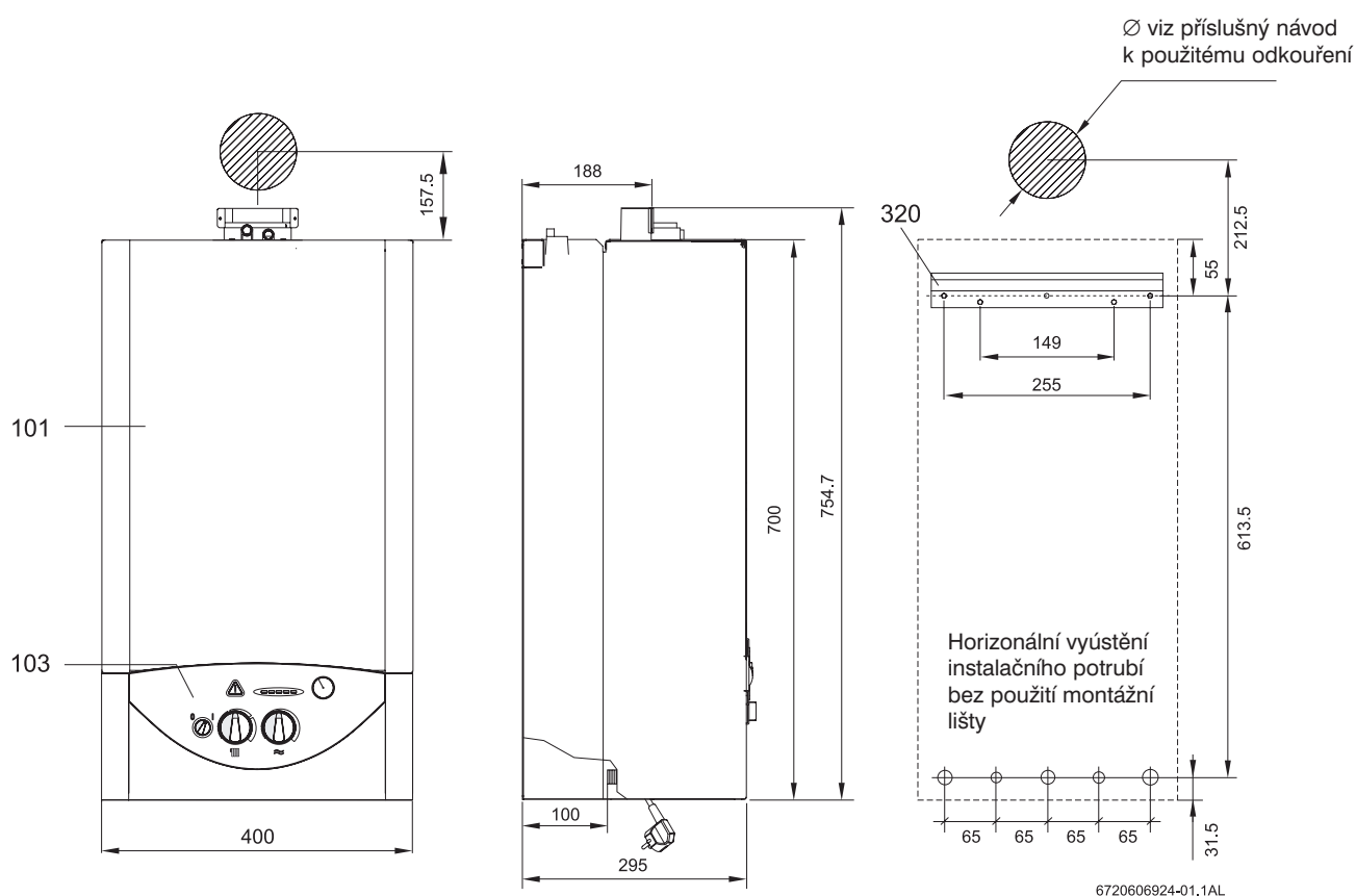
obr. 1 Montážní rozměry - údaje pro otvor odtahu spalin platí pro odkouření AZ 182/184/183/185
