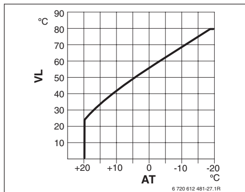
Obr. 14 Základní nastavení otopné křivky pro radiátorové vytápění
