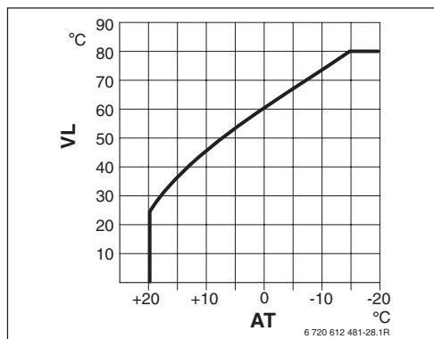
Obr. 15 Základní nastavení otopné křivky pro konvektorové vytápění
