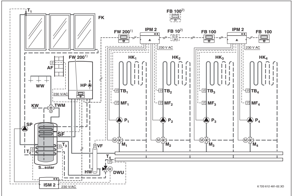
Obr. 4 Zjednodušené schéma zařízení (znázornění způsobu montáže a další možnosti v projekčních podkladech)
