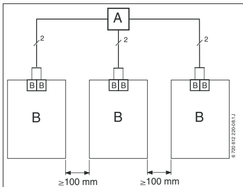
Obr. 10 Připojení sběrnicových spojů přes odbočnou krabici (A)
