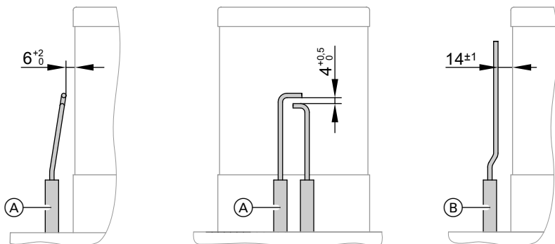
(A) Zapalovací elektrody
