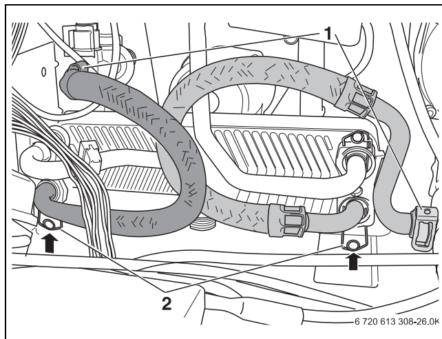
Obr. 17 Montáž hadic
