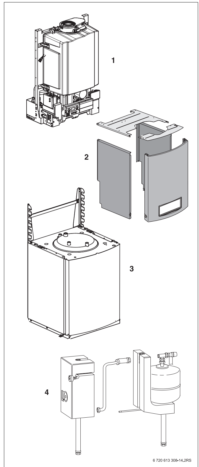
Obr. 3 Rozsah dodávky
