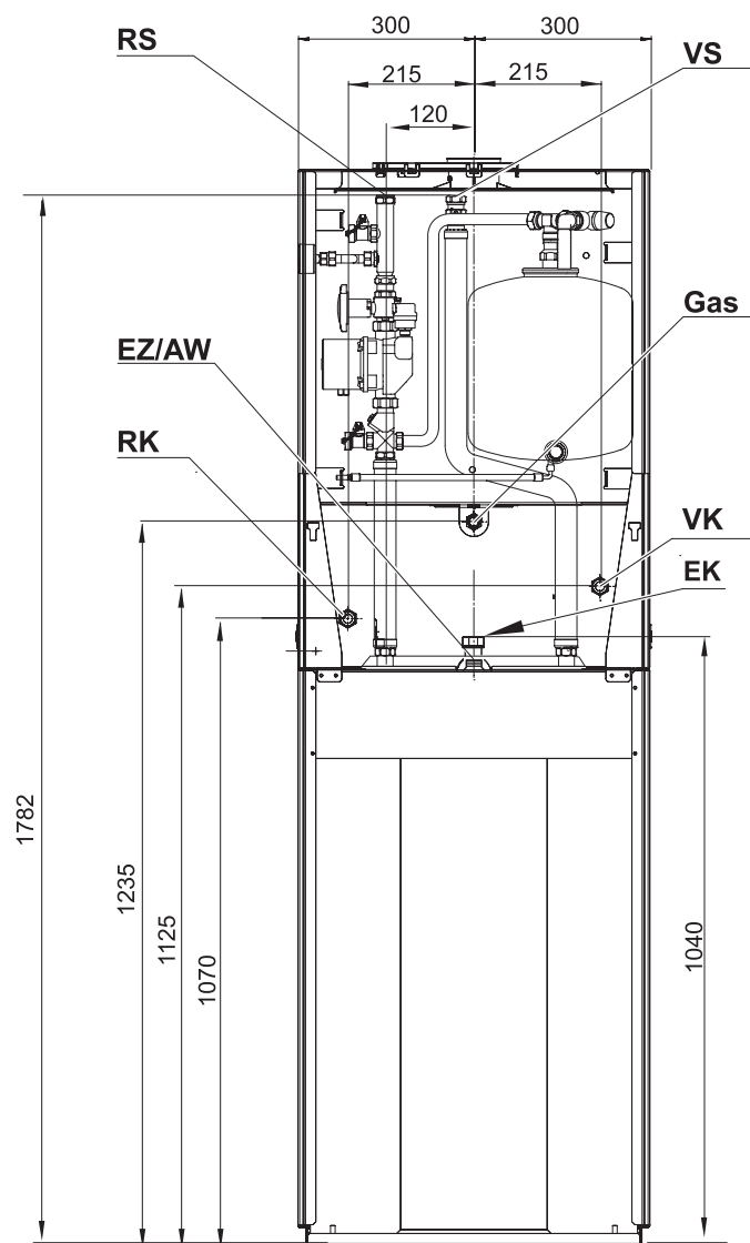
Obr. 6 Rozměry a přípojky pro Logamax plus GB152-24T 170SR (míry jsou uvedeny v mm)
