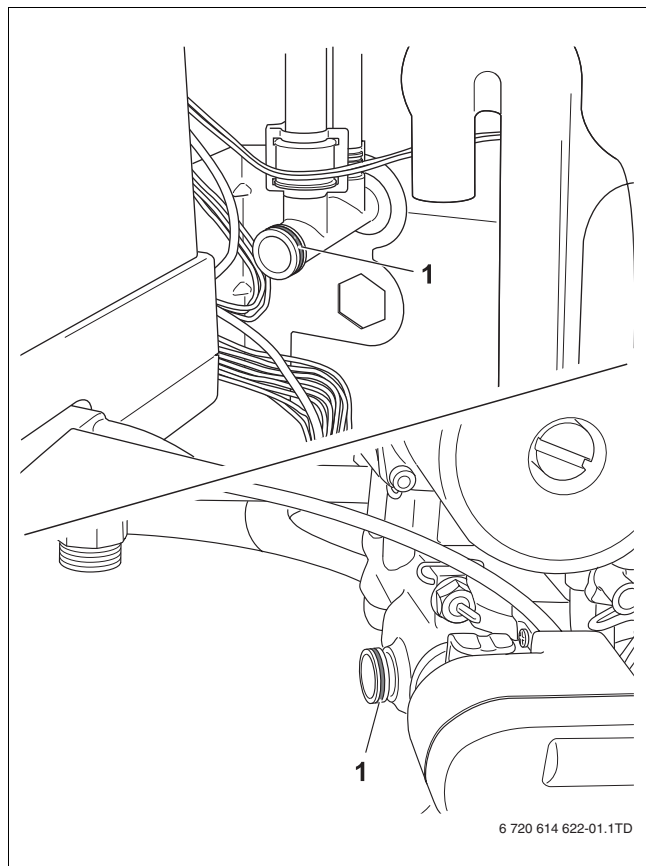
Obr. 12 Montáž O-kroužků
