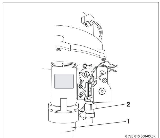
Obr. 80 Plynová armatura
