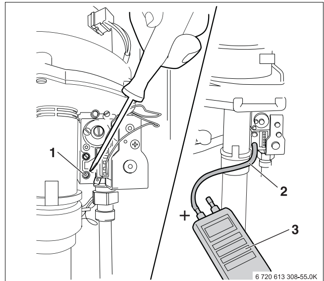
Obr. 68 Měření připojovacího tlaku plynu
