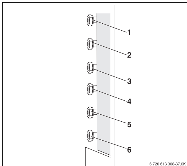
Obr. 38 Připojky u boční přípojovací sady (příslušenství)
