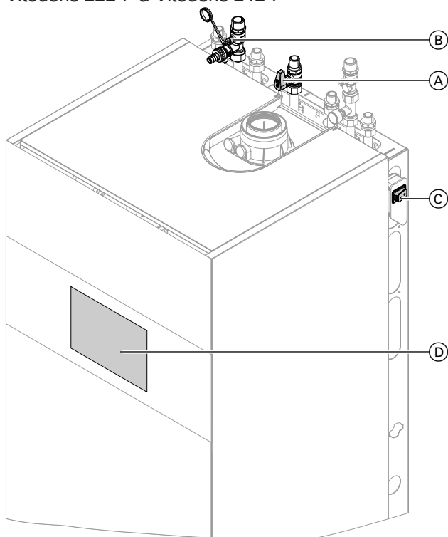
Obr. 15 Příklad s přípojkami nahoru
