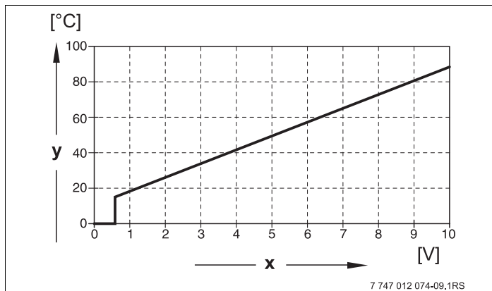
Obr. 1 Vstup 0 – 10 V
