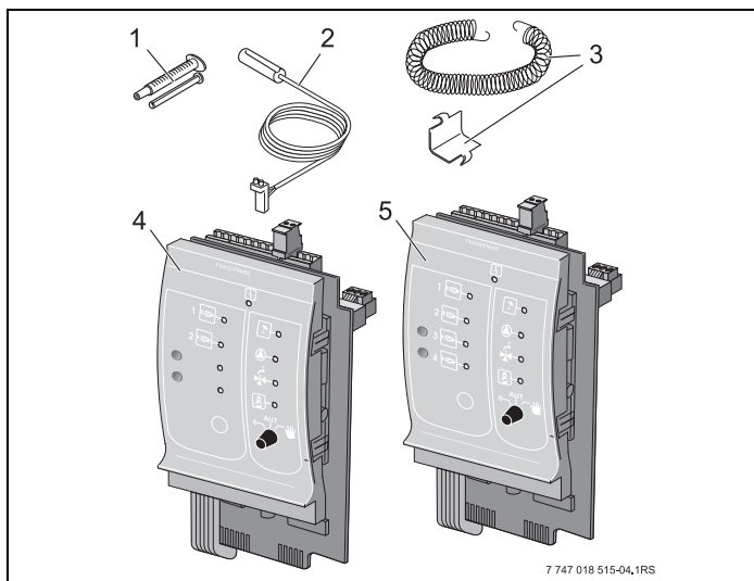
Obr. 4 Rozsah dodávky funkčního modul FM456/FM457
