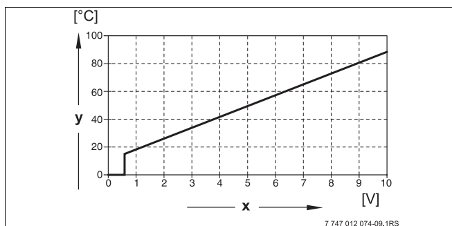
Obr. 10 Vstup 0–10 V
