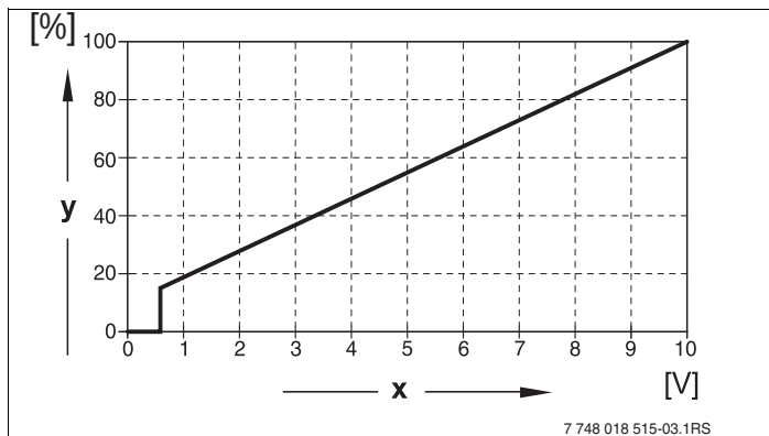
Obr. 2 Vstup 0 – 10 V
