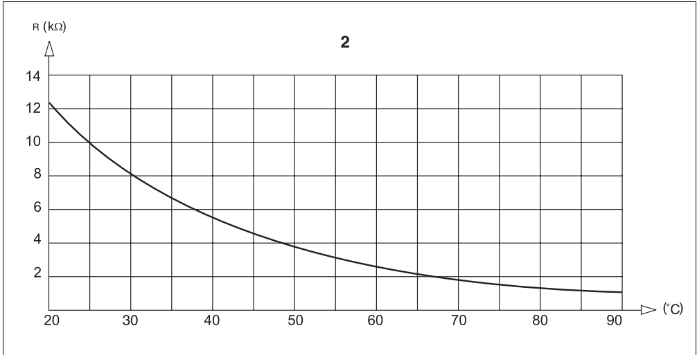
Obr. 14 Charakteristika čidla venkovní teploty a čidla teploty kotlové vody (čidla výstupu zařízení), čidla teploty výstupu, čidla výstupní teploty teplé vody
