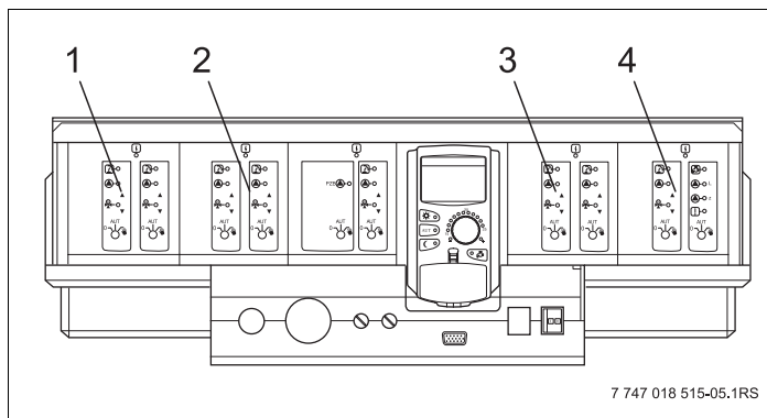
Obr. 5 Přiřazení míst pro zasunutí 1 – 4 (příklad Logamatic 4323)
