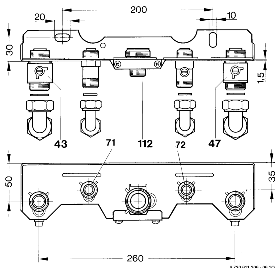
obr. 7 Montážní přípojovací deska
