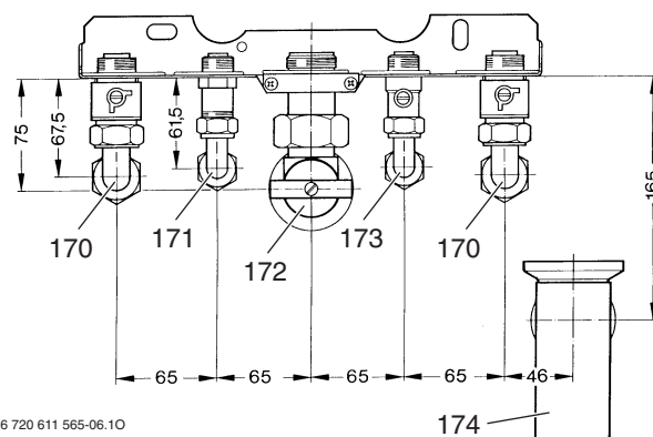
obr. 8 Montážní přípojovací deska s instalací pod omítku (hotově smontována)
