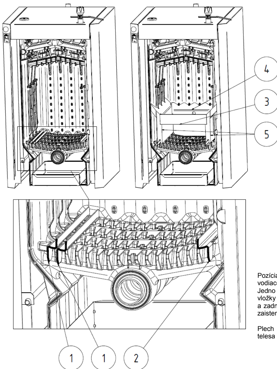
Obr. č. 9 Upresnenie možnosti umiestnenia vodiacich plechov keramik
