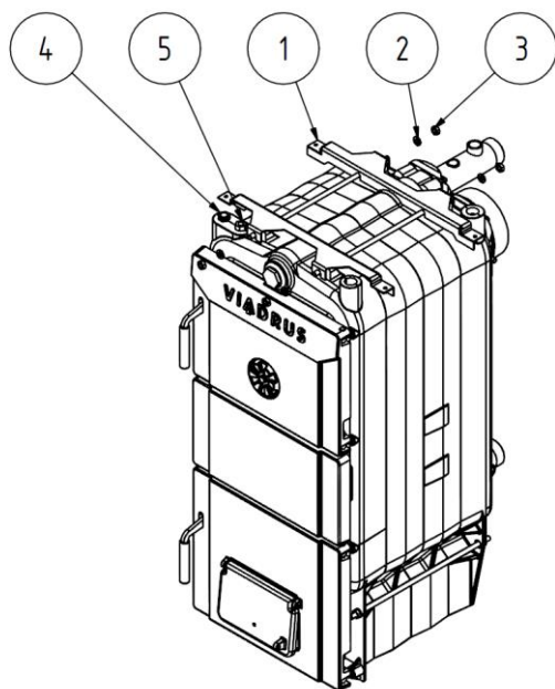
Obr. č. 18 Montáž konzol plášťa
