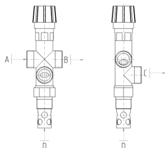
Obr. č. 11 Dvoucestný bezpečnostní ventil DVB 1 - 02
