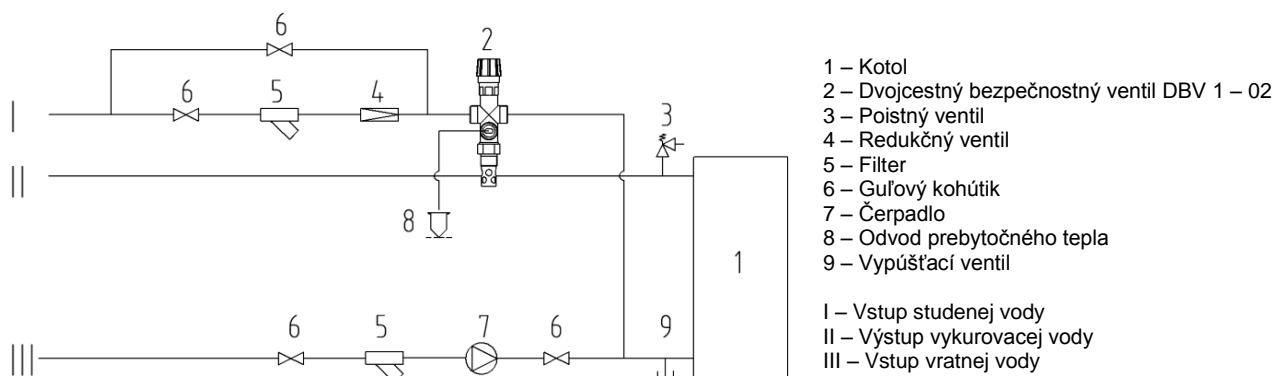
Obr. č. 12 Odporúčaná schéma zapojenia dvojcestného bezpečnostného ventilu DBV 1 – 02
