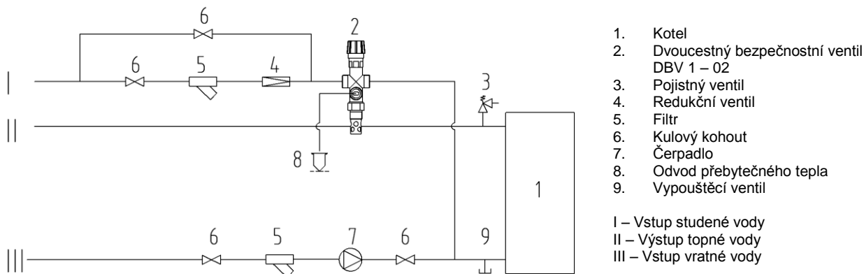
Obr. č. 12 Doporučené schéma zapojení dvoucestného bezpečnostního ventilu DBV 1 - 02
