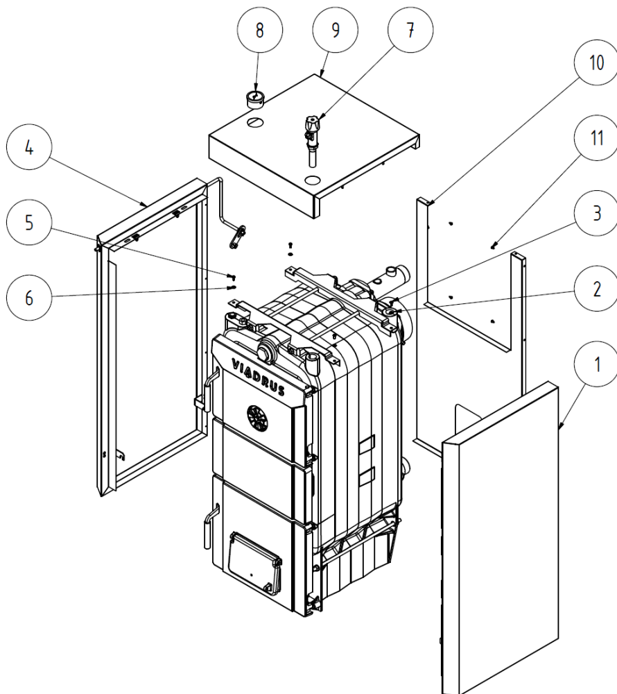
Obr. č. 19 Právý bočný diel plášt'a
