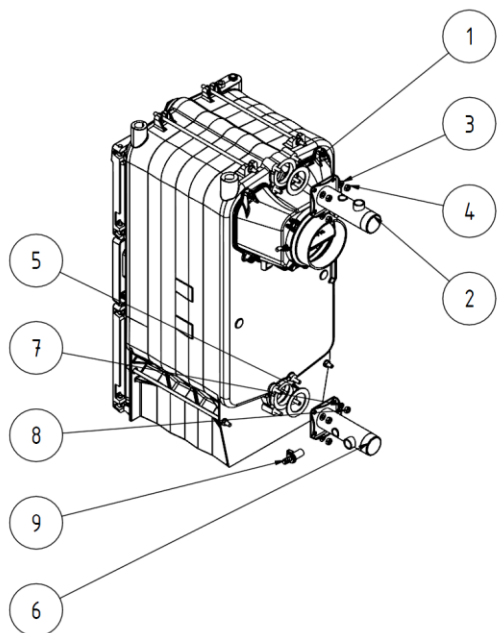
Obr. č. 17 Inštalácia kotlového telesa
