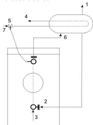
Obr. č. 10 Hydraulická schéma pripojenia dochladzovacej slučky
