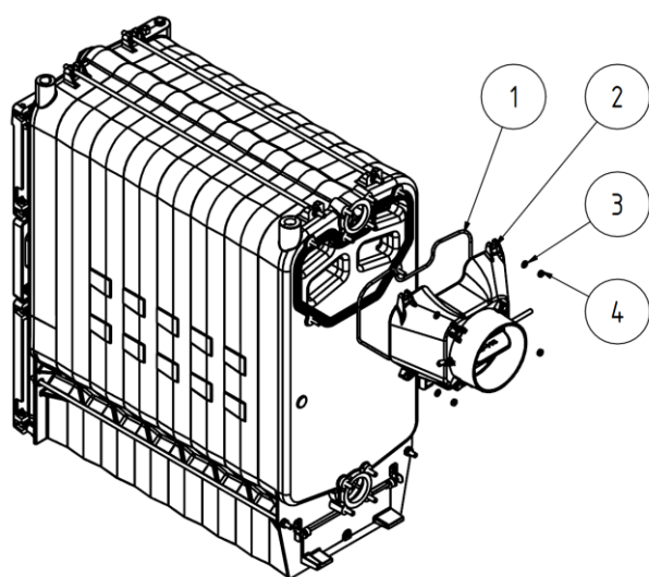
Obr. č. 16 Montáž kouřového nástavce
