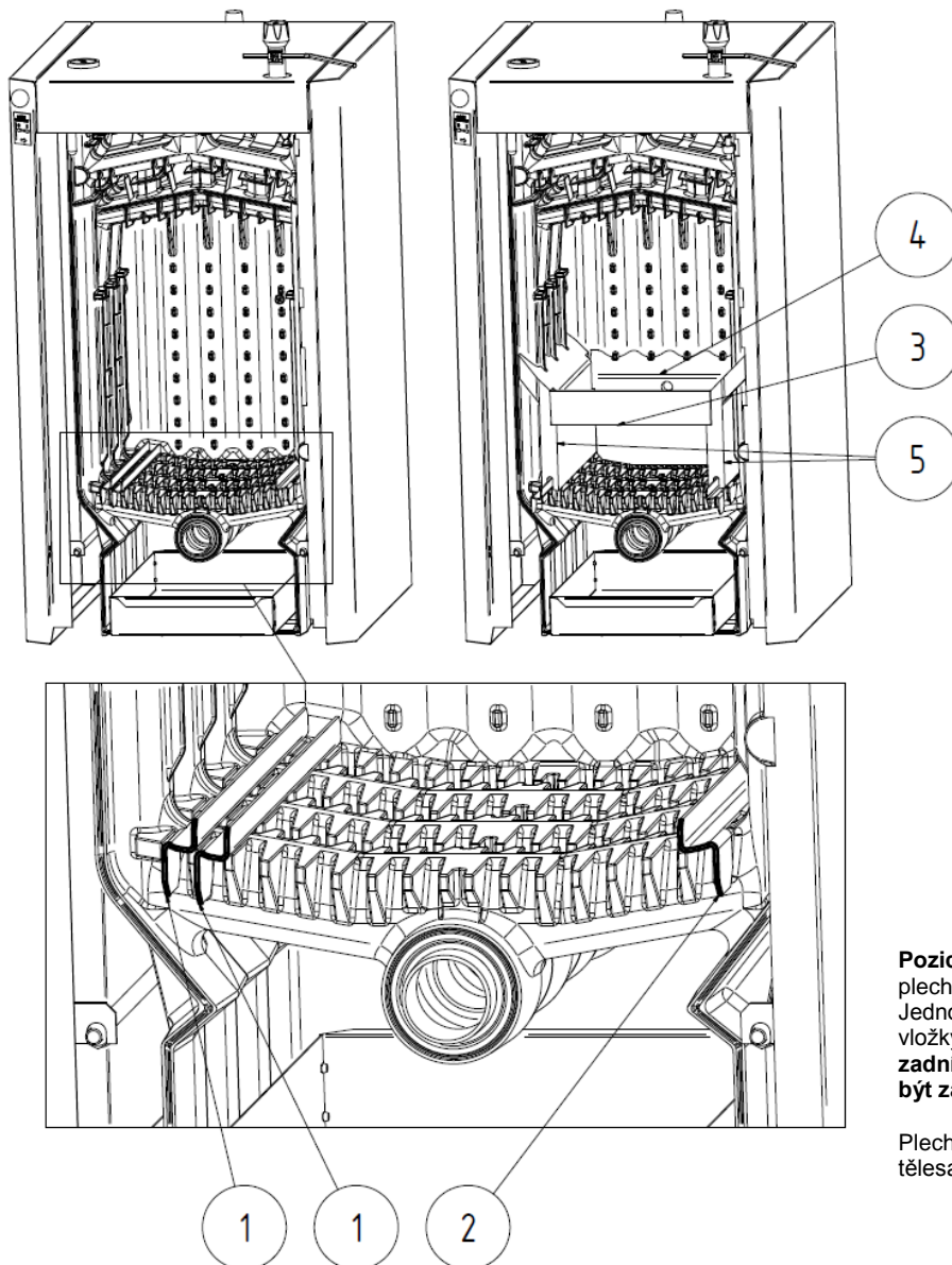
Obr. č. 9 Upřesnění možnosti umístění vodících plechů keramik
