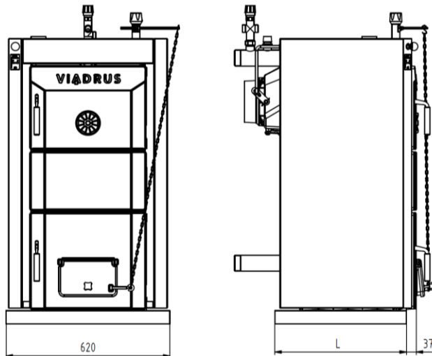
Obr. č. 14 Rozmery podstienky
