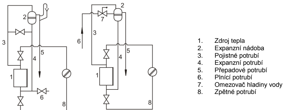
Obr. č. 13 Příklady zapojení otevřených expanzních nádob
