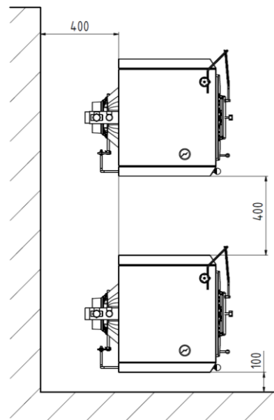
Obr. č. 15 Umiestnenie kotlov v kotelni
