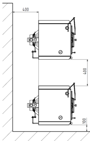
Obr. č. 15 Umístění kotlů v kotelně
