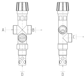
Obr. č. 11 Dvojcestný bezpečnostný ventil DBV 1 – 02
