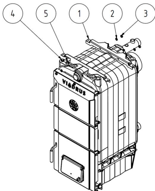
Obr. č. 18 Montáž konzol pláště
