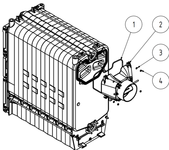
Obr. č. 16 Montáž dymového nadstavca
