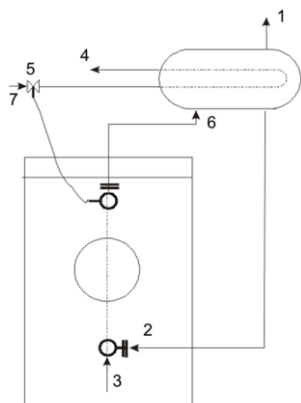
Obr. č. 10 Hydraulické schéma připojení dochlazovací smyčky
