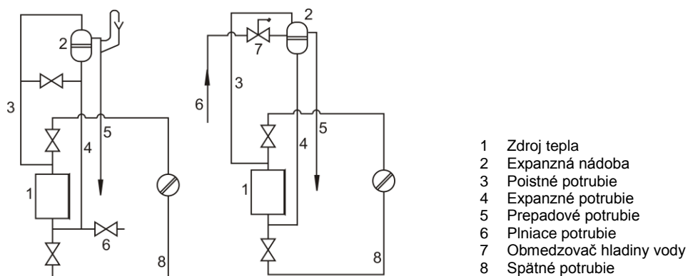
Obr. č. 13 Príklady zapojenia otvorených expanzných nádob
