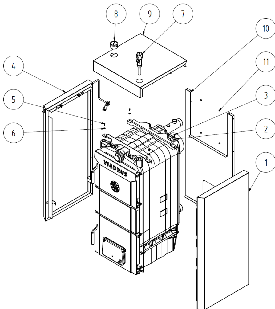
Obr. č. 19 Právý boční díl pláště
