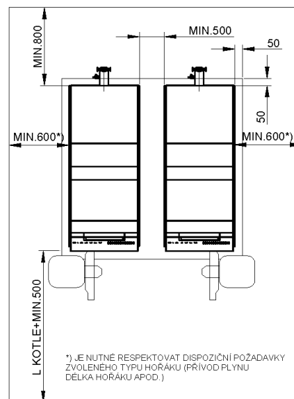
Obr. č. 3 Umístění kotlů v kotelně
