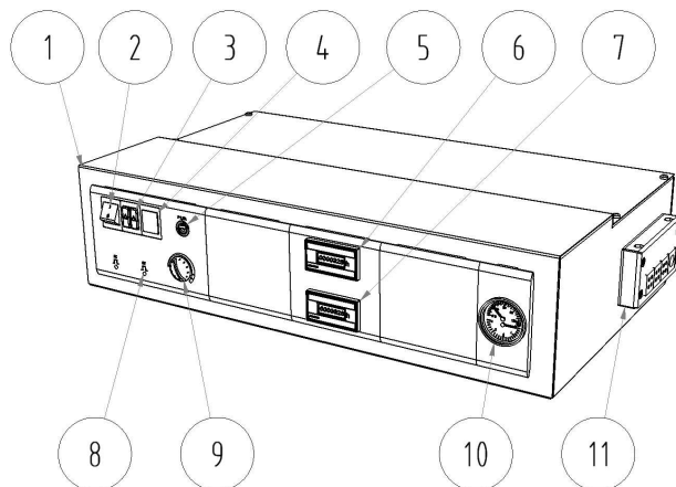
Obr. č. 12 Sestava elektropanelu
