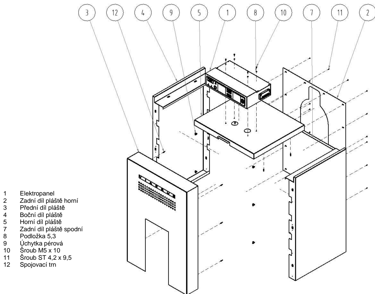
Obr. č. 10 Montáž opláštění
