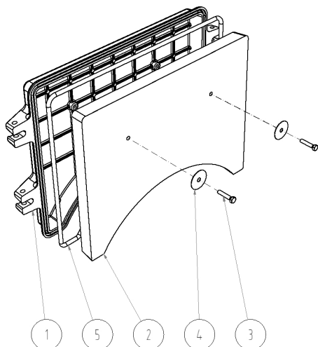
Obr. č. 7 Montáž uzavěrné desky
