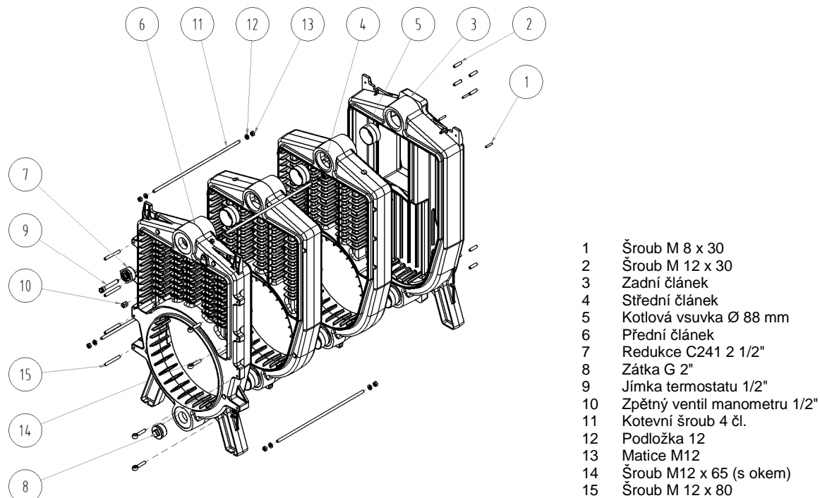
Obr. č. 4 Montáž kotlového tělesa 4 čl. velikosti
