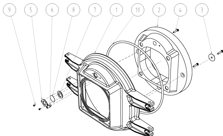
Obr. č. 6 Montáž hořákové desky
