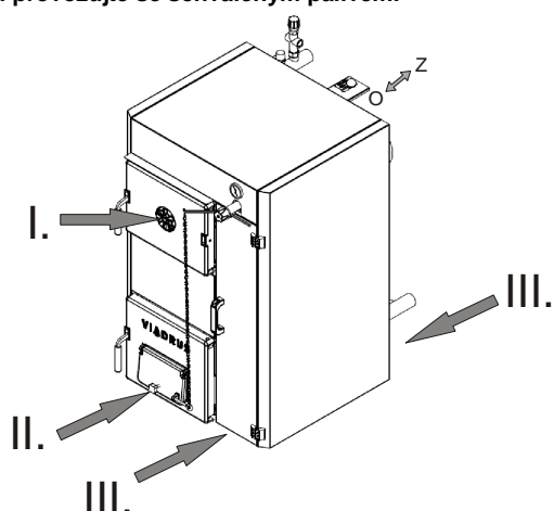
Obr. č. 18 Přívod vzduchů do kotle
