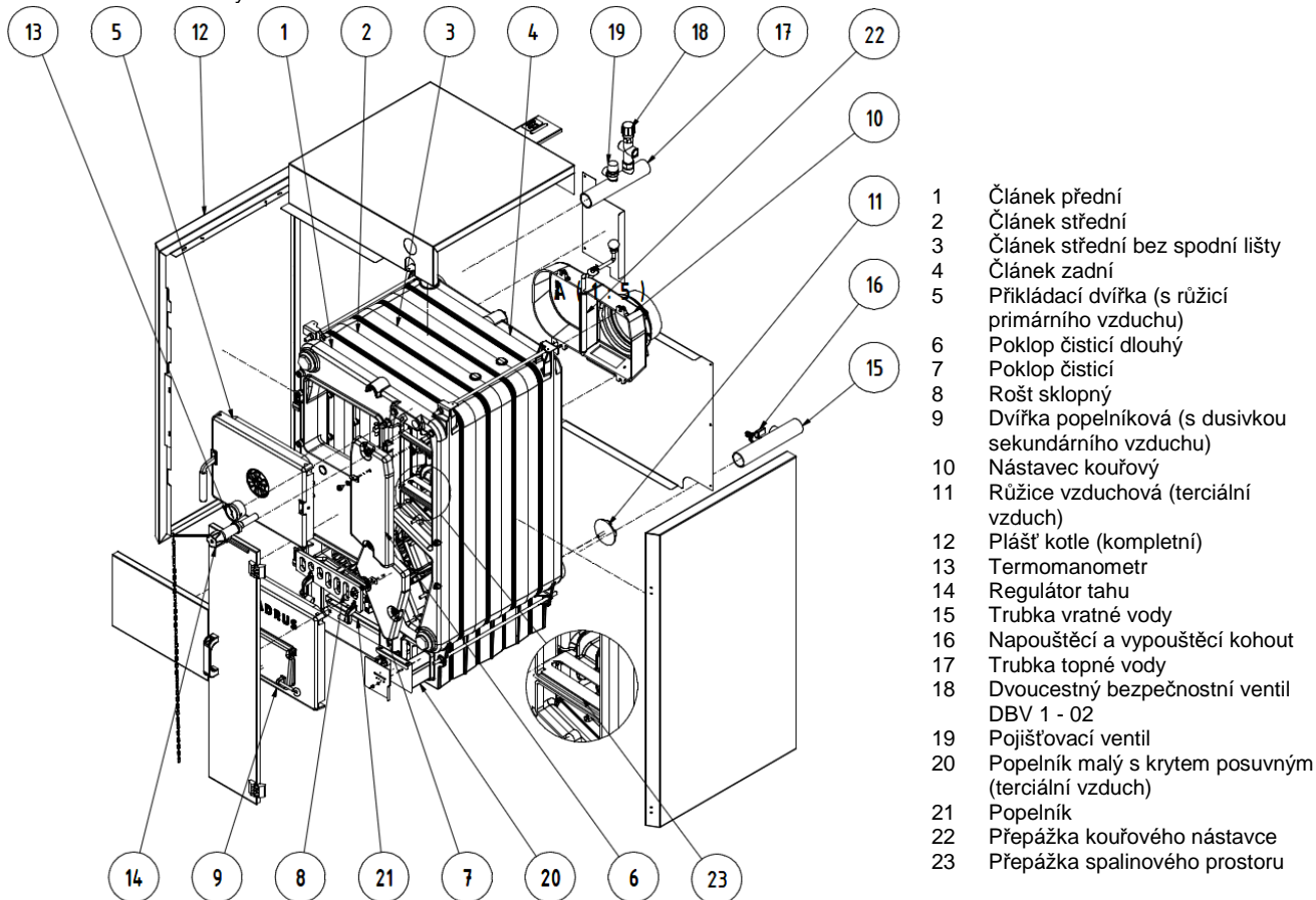
Obr. č. 3 Hlavní části kotle
