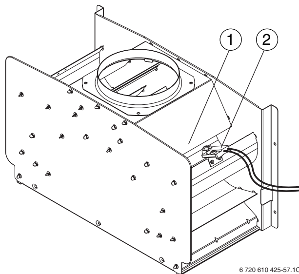
obr. 60 Čidlo hlídače odtahu spalin na přerušovači tahu
