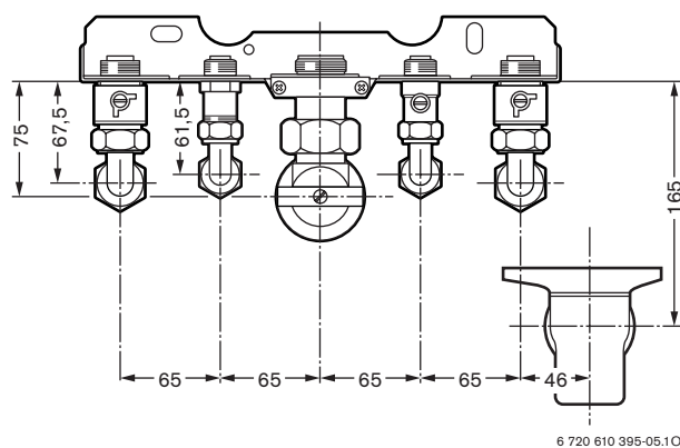
obr. 8 Montážní připojovací deska
