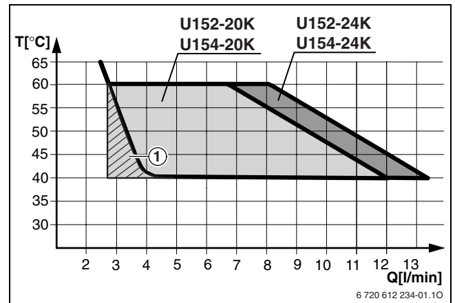
Obr. 9 Graf vstupní teploty studené vody +15 °C
