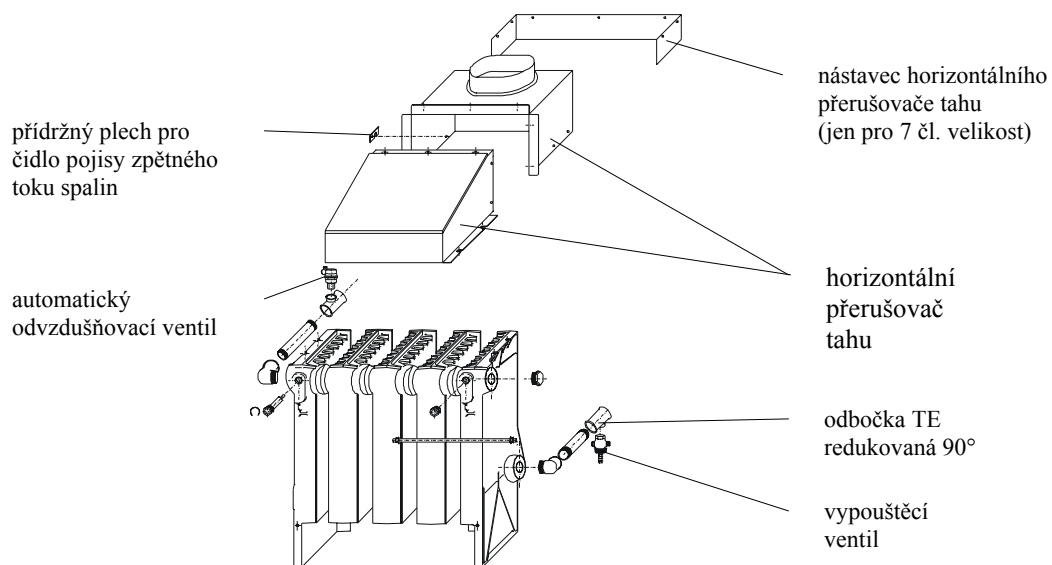
Obr. č. 18 Napojení na otopný systém a montáž přerušovače tahu
