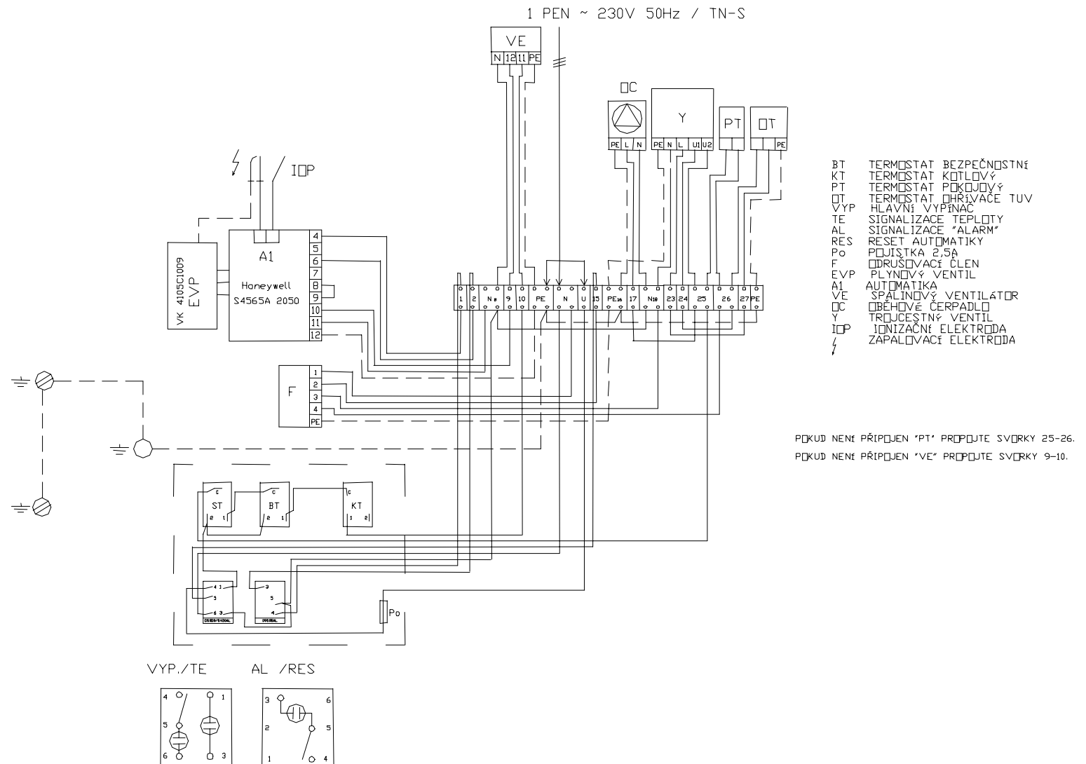
Obr.č. 5 Elektrické schéma kotle VIADRUS G 27 ECO GL (XZ010, XZ011, XZ012, XZV10, XZV11, XZV12) s jednodupňovým plynovým ventilem v kombinaci s prostorovým termostatem Honeywell K42007508-001 nebo program. regulátorem Honeywell CM 27
