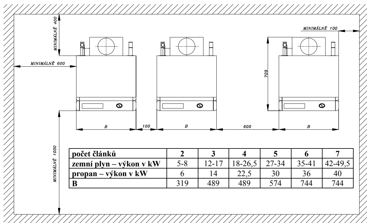
Obr. č. 17 Umístění kotlů v kotelně
