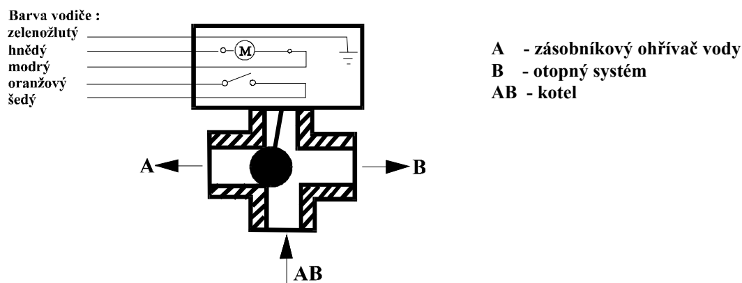
Obr. č. 21 Trojcestný ventil Honeywell V 4044F
