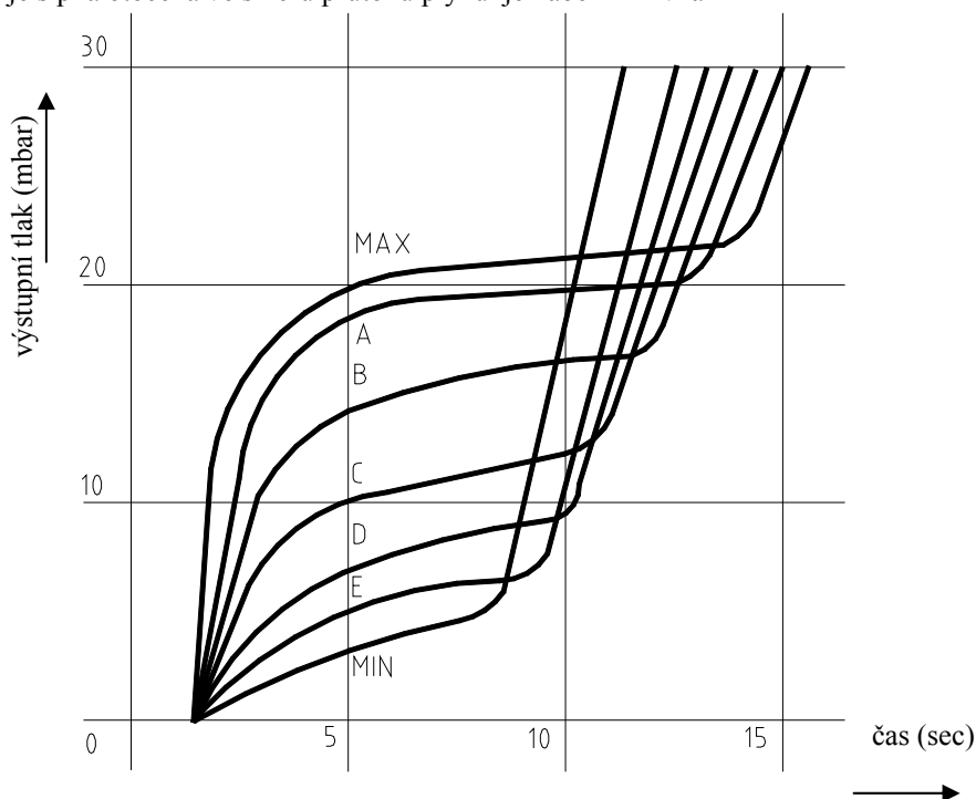
Obr. č. 27 Otevírací charakteristiky hlavního ventilu
