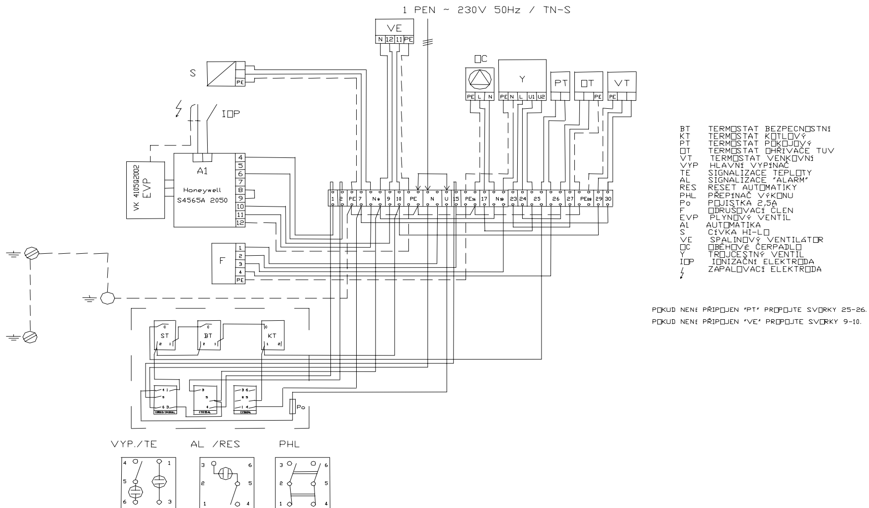
Obr. č. 3 Elektrické zapojení kotle VIADRUS G 27 ECO GL (XZ020, XZ021, XZ022, XZV20, XZV21, XZV22) s dvoustupňovým plynovým ventilem v kombinaci s prostorovým termostatem Honeywell K42007508-001 nebo programovatelným regulátorem Honeywell CM 27
