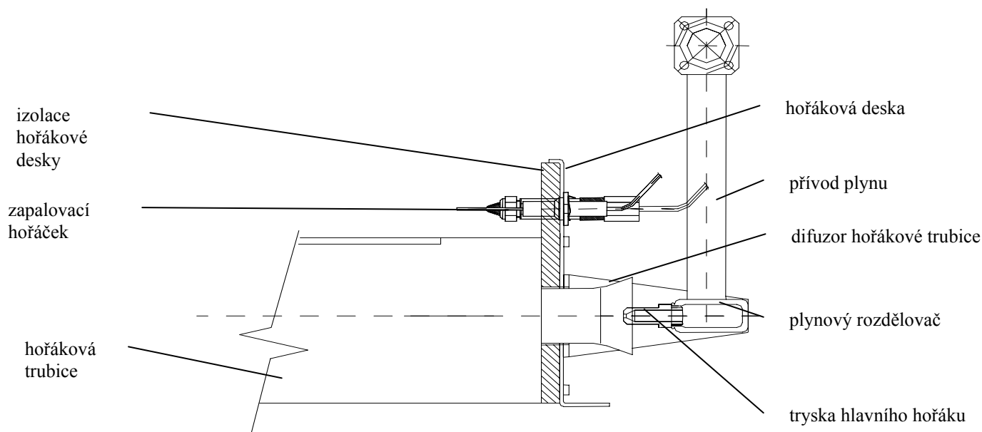
Obr. č. 15 Umístění zapalovacího hořáčku nad hořákem
