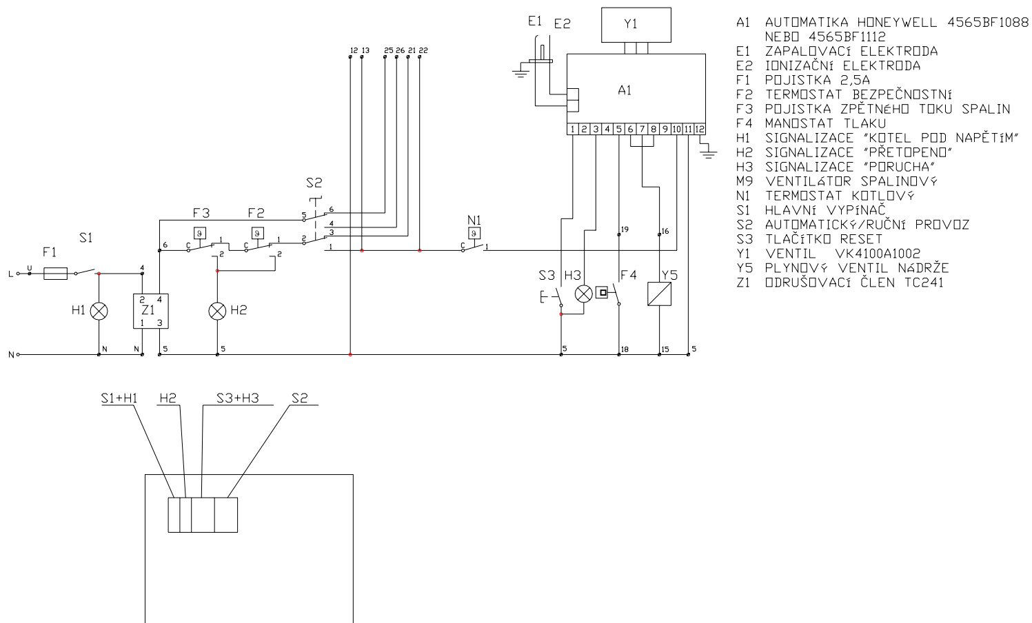
Obr. č. 11 Obvodové schéma kotle G27 ECO GLX pro palivo propan
