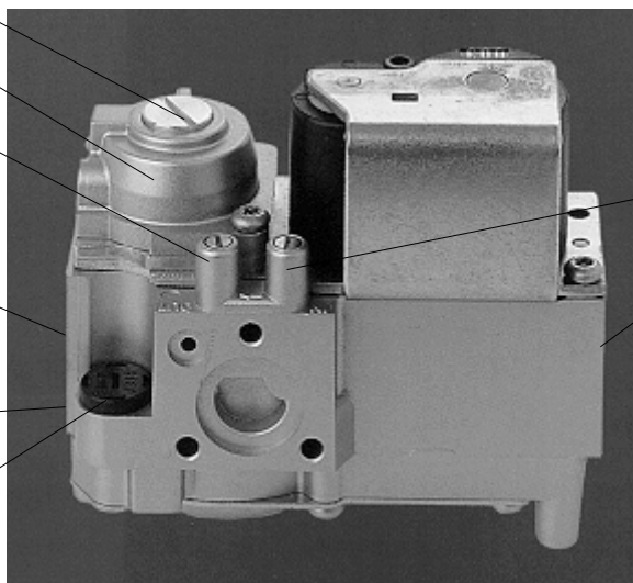
Obr. č. 26 Plynový ventil Honeywell VK 4105 C 1009 a VK 4100 A 1002
