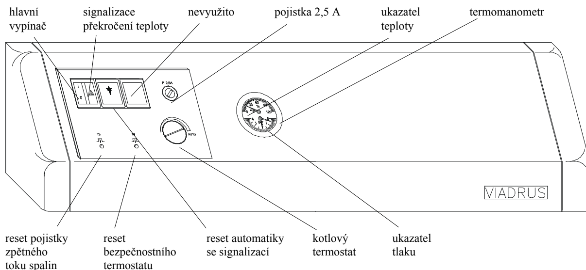
Obr. č. 29 Ovládací panel kotle VIADRUS G 27 ECO GL (XZ010, XZ011, XZ012, XZV10, XZV11, XZV12, XP010, XP011, XP012, XPV10, XPV11, XPV12) s jednostupňovým plynovým ventilem a vybaveného prostorovým termostatem Honeywell K42007508-001 nebo programovatelným regulátorem Honeywell CM 27
