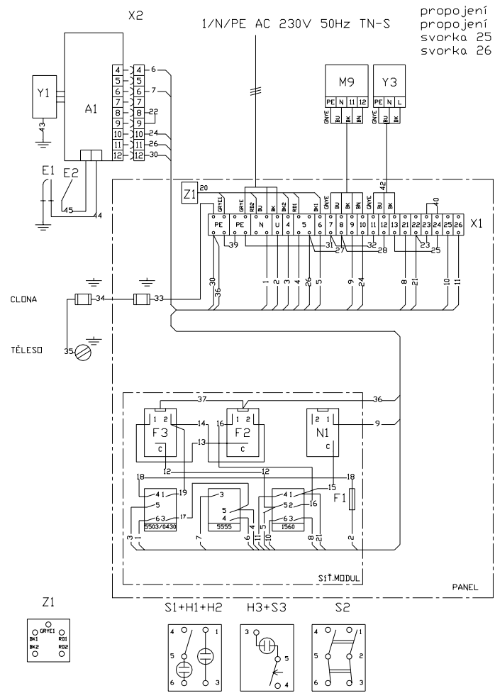
Obr. č. 8 Elektrické schéma kotle G27 ECO GLX pro palivo zemní plyn
