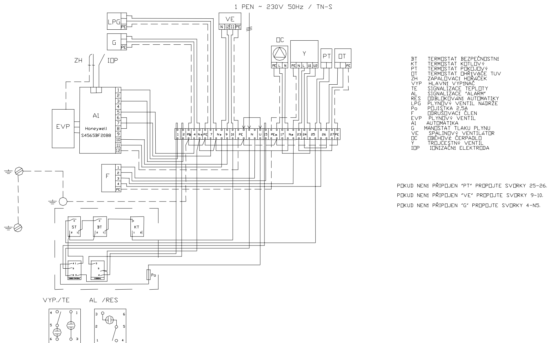
Obr.č. 7 Elektrické schéma kotle VIADRUS G 27 ECO GL(XP010, XP011, XP012, XPV10,XPV11,XPV12) s jednoduší plynovým ventilem v kombinaci s prostorovým termostatem Honeywell K42007508-001 nebo programovatelným regulátorem Honeywell CM 27
