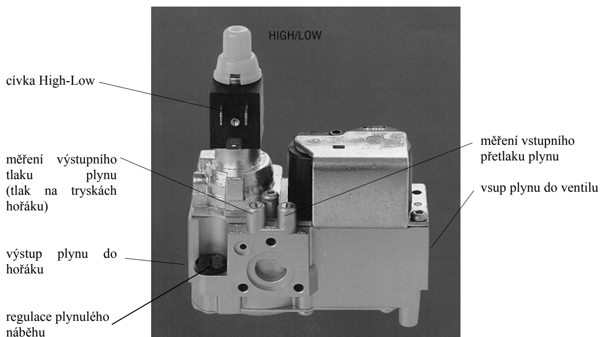
Obr. č. 25 Plynový ventil Honeywell VK 4105 Q 2002
